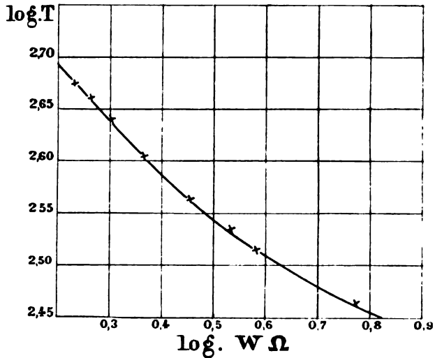
Fig. 1 Eisenglanz von Onro Preto. Stab \perp zur Achse.
